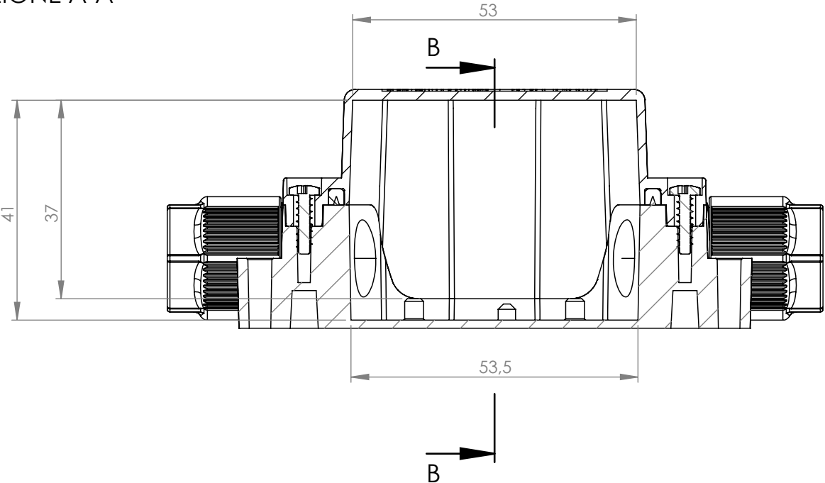
SEZIONE A-A
